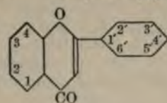
Flavone.
